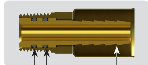
Vue en coupe d'un raccord
